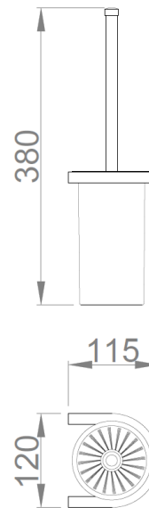
РАЗМЕРЫ В мм
